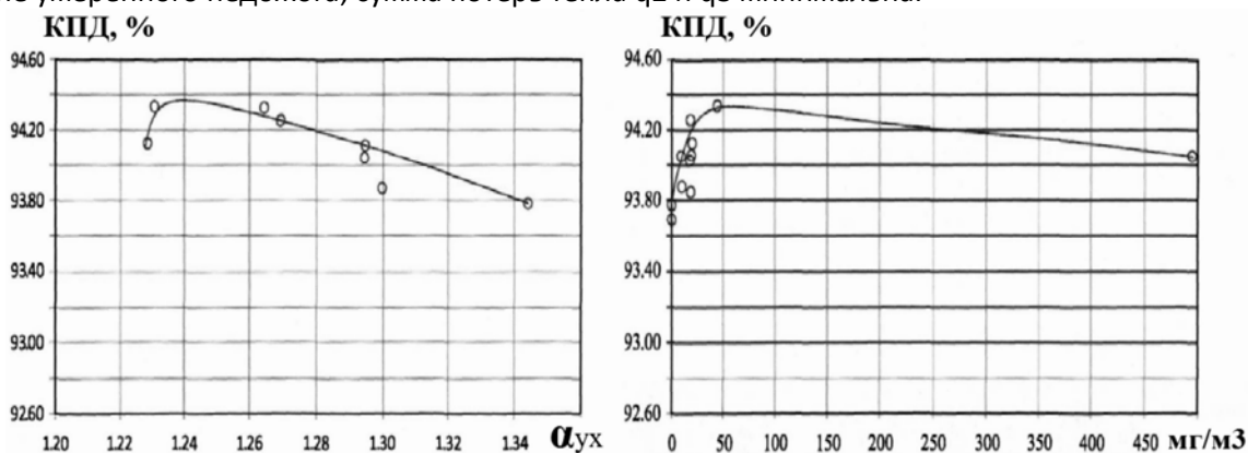
Изменение КПД котла ТГМ-84Б (Е-420-140ГМ) при сжигании природного газа, D=370-380 т/ч. А-влияние избытка воздуха; Б-влияние концентрации СО в дымовых газах
